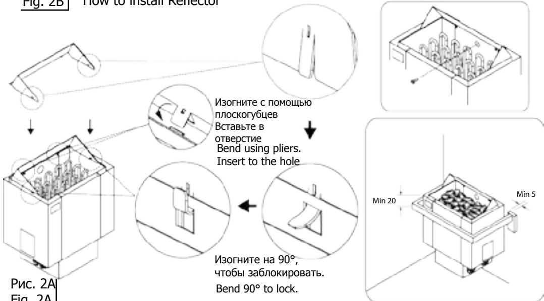
Рис. 2B) Прикрепление отражателя Fig. 2B) How to install Reflector
